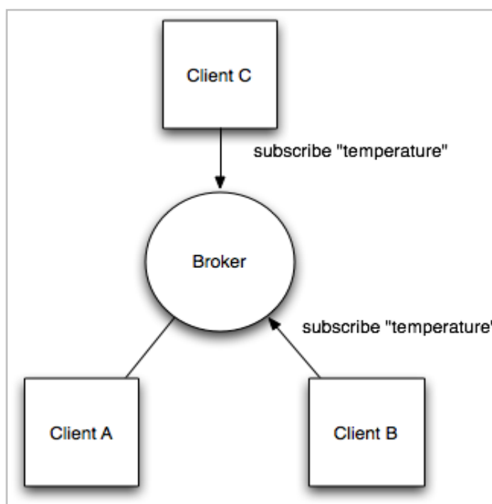
Figura 2: Estrutura de assinatura MQTT.
